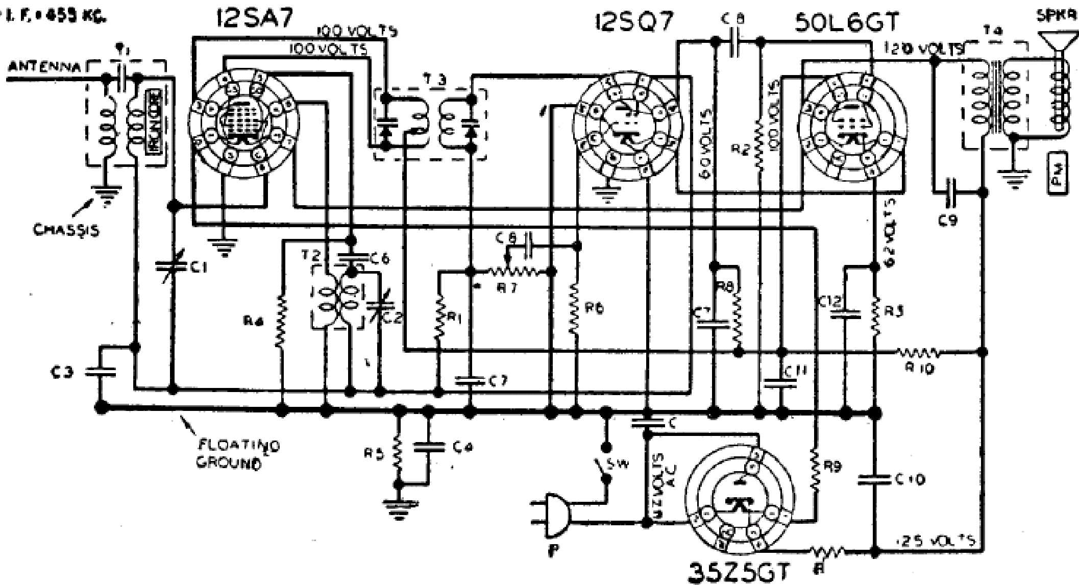
Fig. 6.1. - Esempio di minuscola supereterodina americana.
